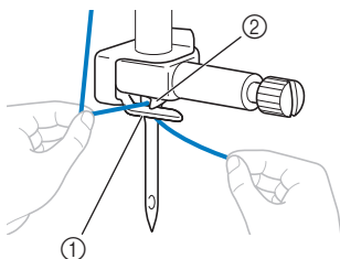
① Prowadnik nici igielnicy ② Haczyk
